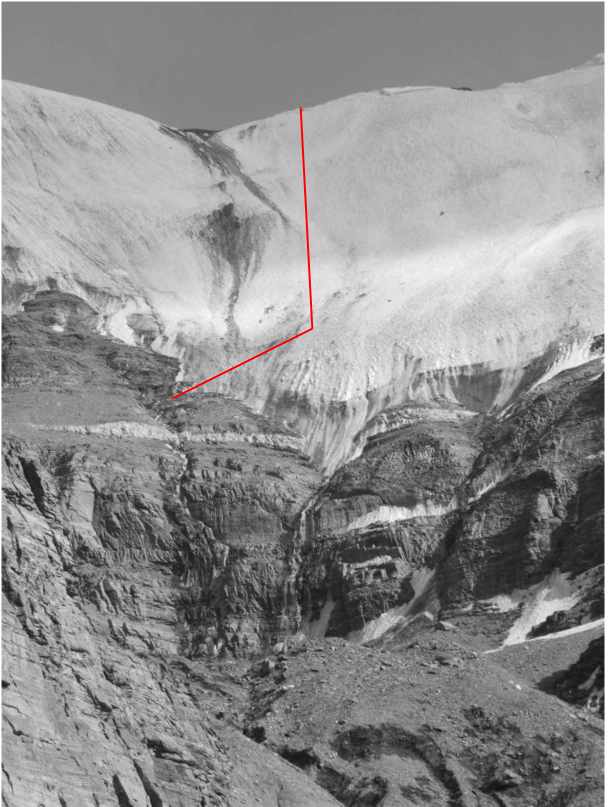
DIULFERIS 45° LEDO ŠLAITU: 6 VIRVĒS x 50 m + 2 VIRVĒS HORIZONTALIŅU TURĒKLU
