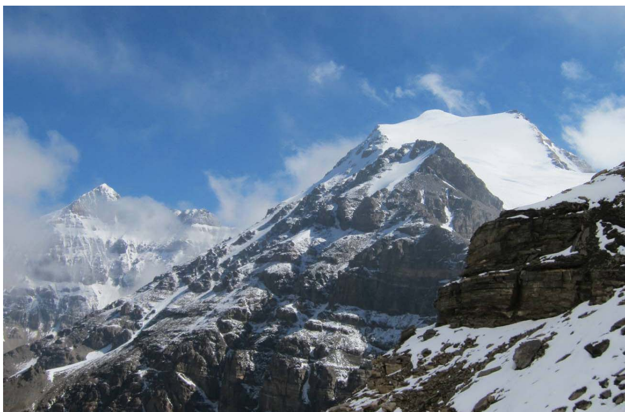
DARIAUS IR GIRĖNO (dešinėje) IR LITUANIKOS (kairėje, tolimoje) VIRŠŪNĖS NUO ŠACHDAROS KALNAGŪBRIO PIETINĖS KETEROS
